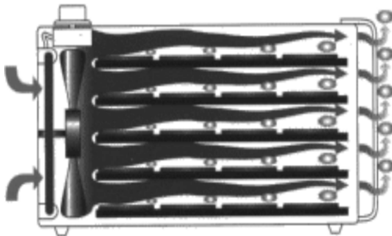
Принцип роботи Турбо-сушок з паралельним обдуванням
