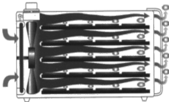
Принцип работы Турбо-сушек с параллельным обдувом
