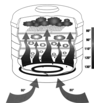
Стандартный принцип работы круглой сушки без конвекции.
